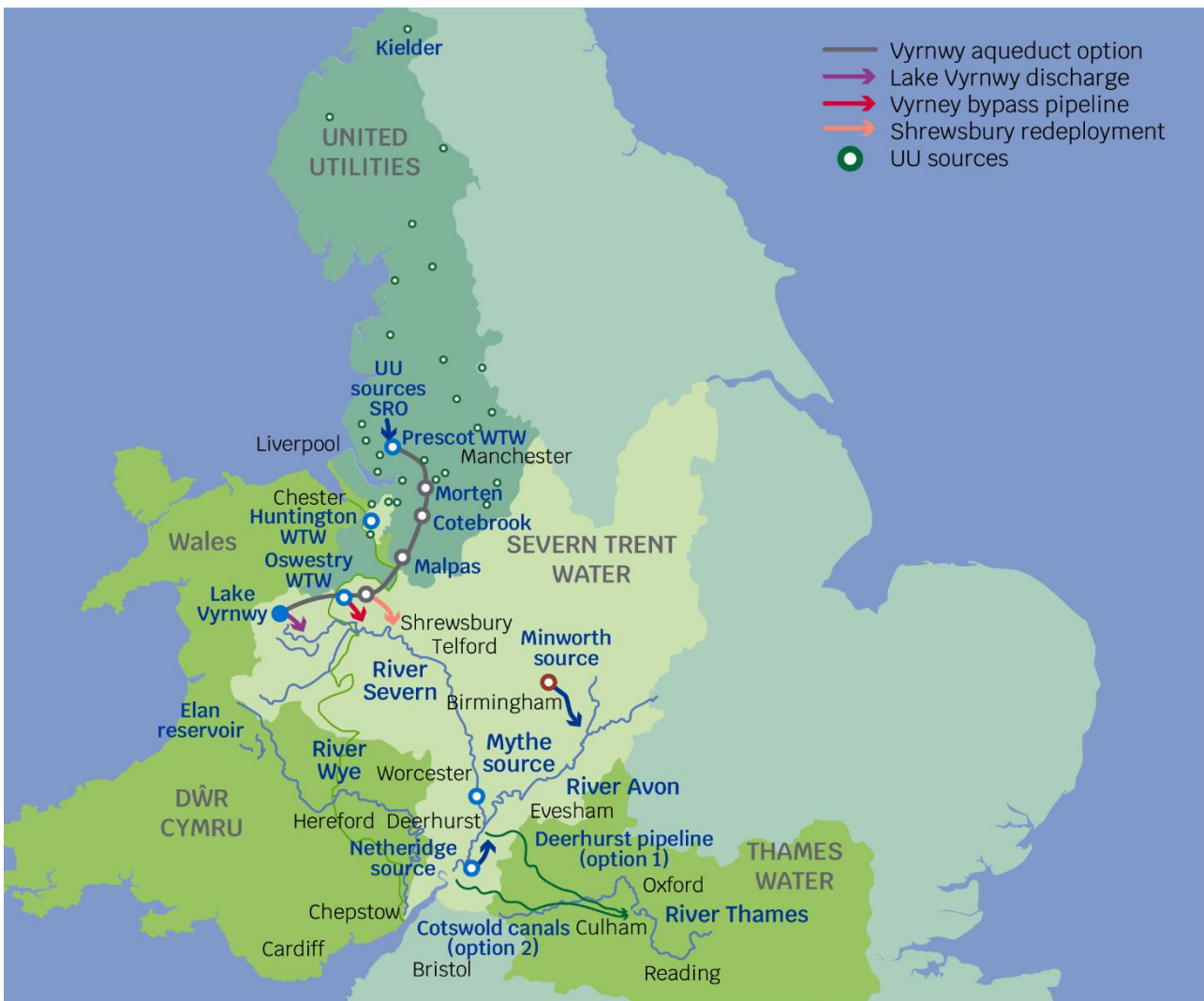
Ffigur 1 Sgematig datrysiad UUS
